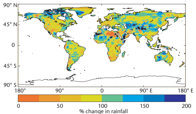
Rainfall anomalies for 2003, relative to 1961–90. Raw data provided by Deutscher Wetterdienst
